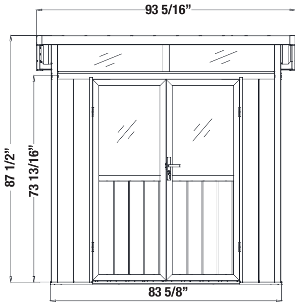
EN FRONT ELEVATION
