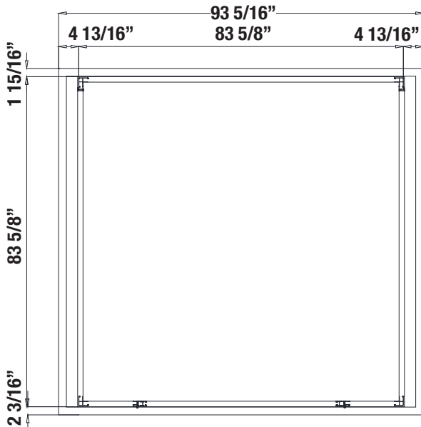
EN TOP VIEW
