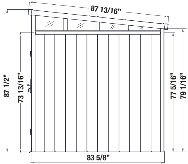
RIGHT ELEVATION
