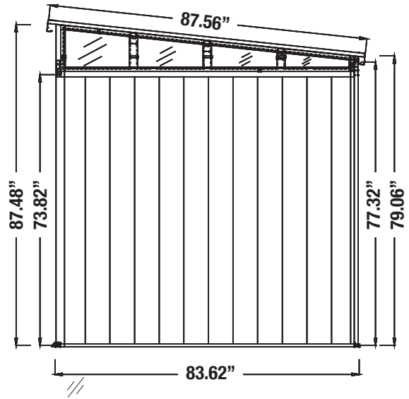
RIGHT ELEVATION ÉLÉVATION DE LA DROITE
