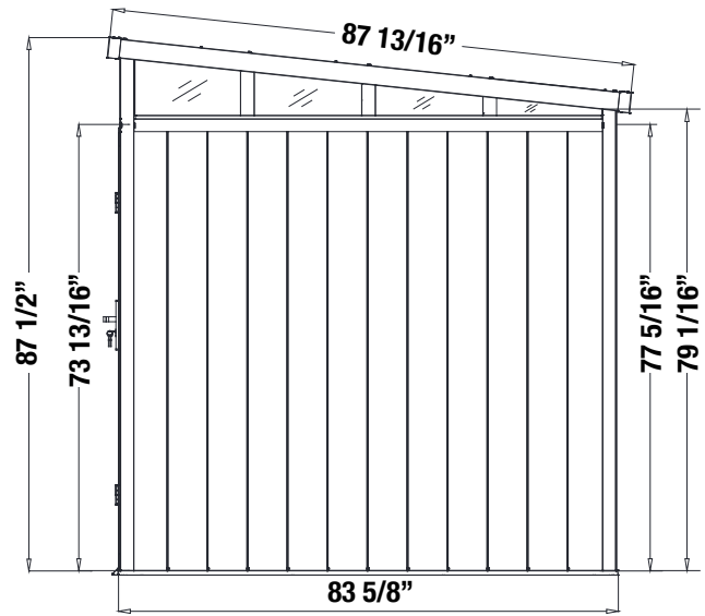
RIGHT ELEVATION ÉLÉVATION DE LA DROITE
