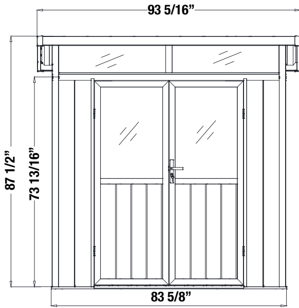
EN FRONT ELEVATION FR ÉLÉVATION DE LA FAÇADE
