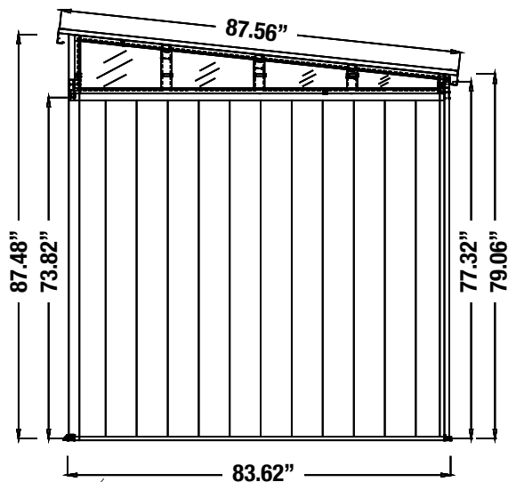
RIGHT ELEVATION ÉLÉVATION DE LA DROITE
