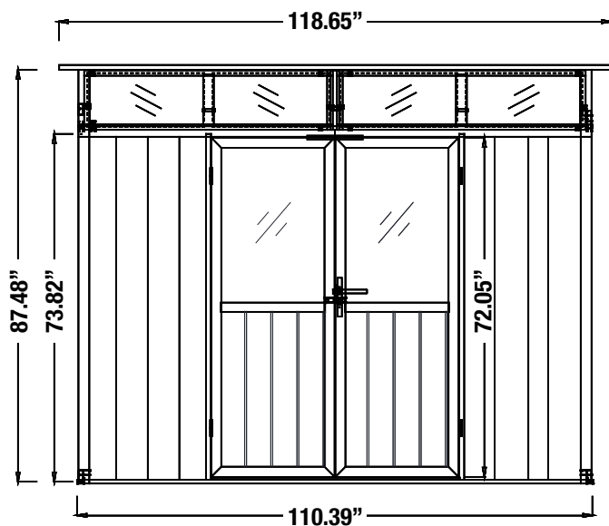
EN FRONT ELEVATION FR ÉLÉVATION DE LA FAÇADE
