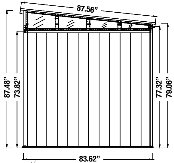
SIDE VIEW VUE LATÉRALE
