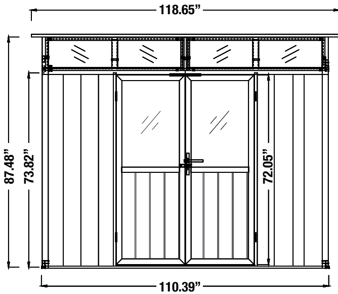
EN FRONT VIEW FR VUE FRONTALE
